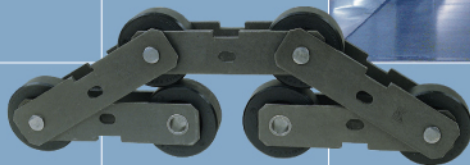
Passenger conveyor chains Ketten für Fahrsteige
